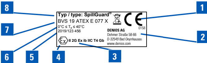
III. 4: Rappresentazione schematica CE
